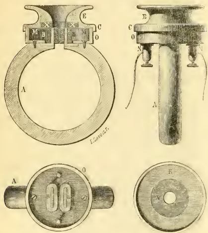
FIG. 4.—Ader's telephone à surexcitation .
