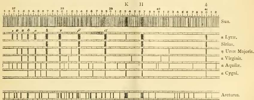
FIG. 43.—Stellar spectra (Huggins).
